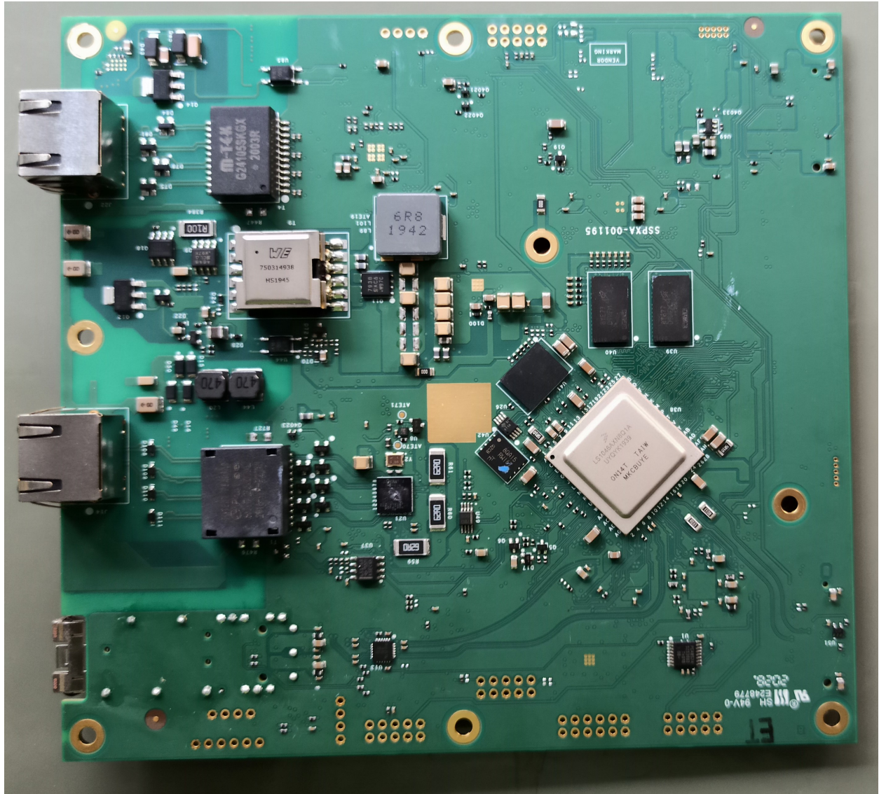
V3000 SSAXA-001000 PCBA Top View
