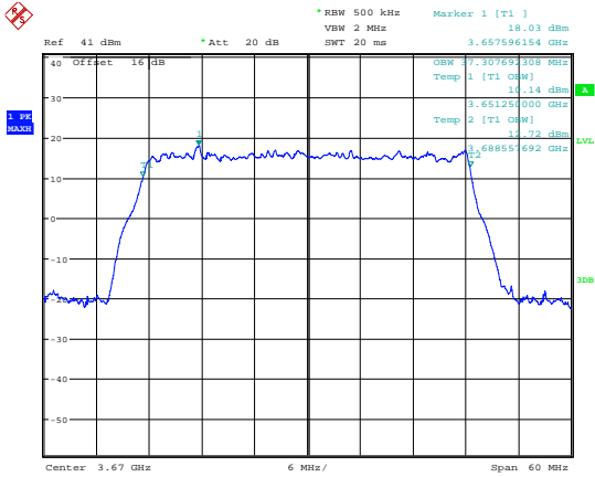
99 % Bandwidth; QPSK; 3670 MHz; MIMO A.
