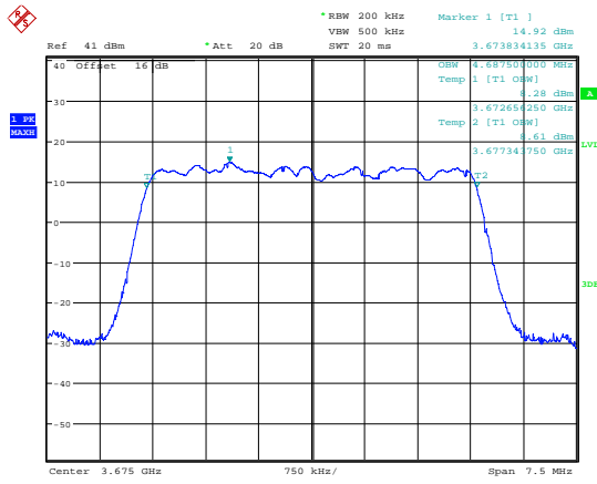
Date: 7.JUL.2018 19:02:14 99 % Bandwidth QPSK; 3675 MHz; MIMO A.
