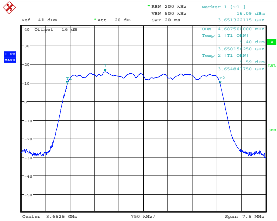
99 % Bandwidth; QPSK; 3652.5 MHz; MIMO A.
