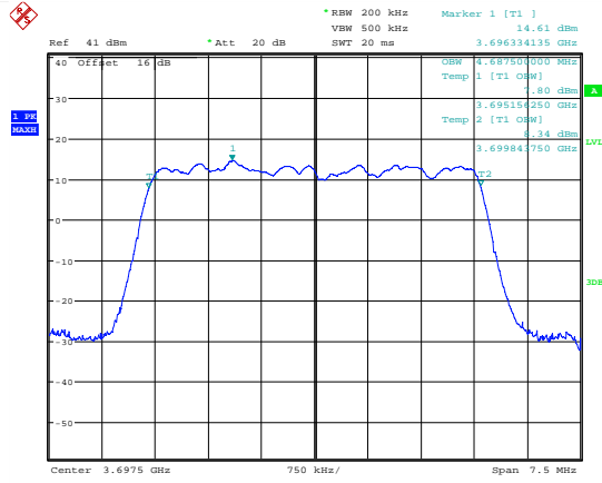
Date: 7.JUL.2018 19:06:15 99 % Bandwidth QPSK; 3697.5 MHz; MIMO B.
