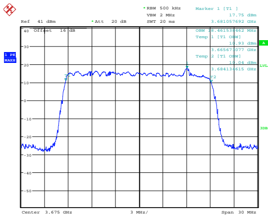
Date: 7.JUL.2018 17:19:24 99 % Bandwidth; QPSK; 3675 MHz; MIMO A.
