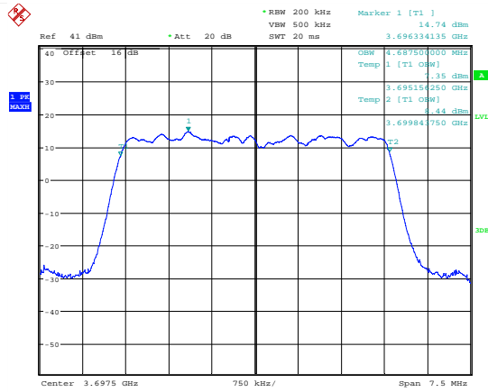
Date: 7.JUL.2018 19:06:15 99 % Bandwidth QPSK; 3697.5 MHz; MIMO B.
