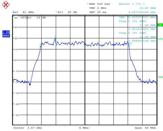
99 % Bandwidth; QPSK; 3670 MHz; MIMO A.
