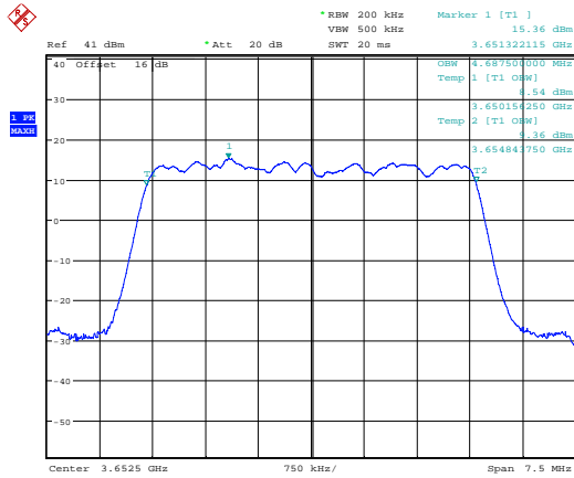
99 % Bandwidth QPSK; 3652.5 MHz; MIMO A.
