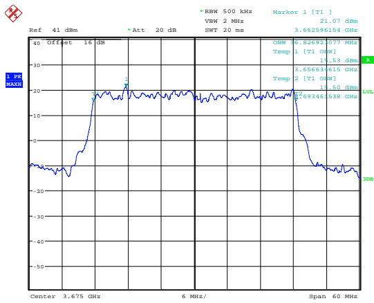
Date: 7.JUL.2018 19:54:20 99 % Bandwidth; QPSK; 3675 MHz; MIMO A.
