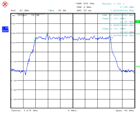
Date: 7.JUL.2018 19:52:56 99 % Bandwidth; QPSK; 3675 MHz; MIMO A.
