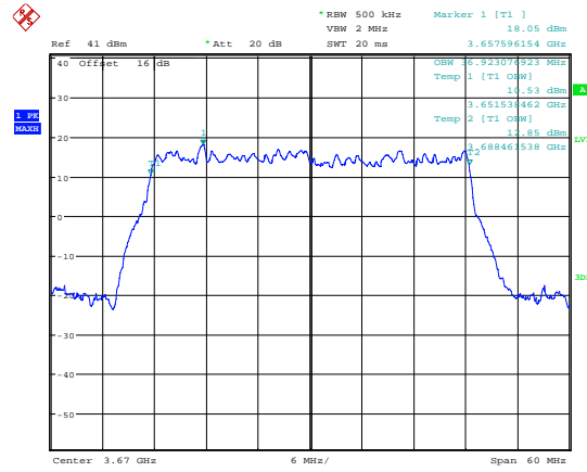
99 % Bandwidth; QPSK; 3670 MHz; MIMO B.
