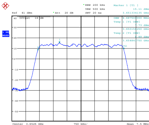
99 % Bandwidth; QPSK; 3652.5 MHz; MIMO A.
