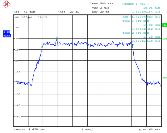
Date: 7.JUL.2018 19:50:09 99 % Bandwidth; QPSK; 3675 MHz; MIMO B.
