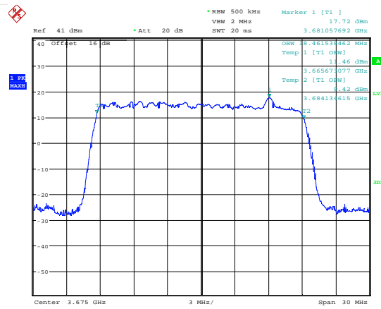
Date: 7.JUL.2018 17:22:21 99 % Bandwidth; QPSK; 3675 MHz; MIMO B.
