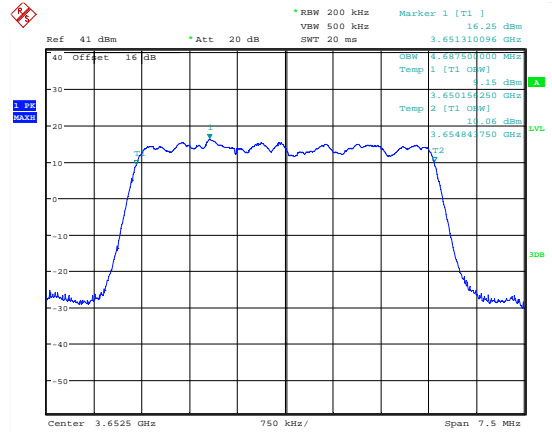
99 % Bandwidth; QPSK; 3652.5 MHz; MIMO B.
