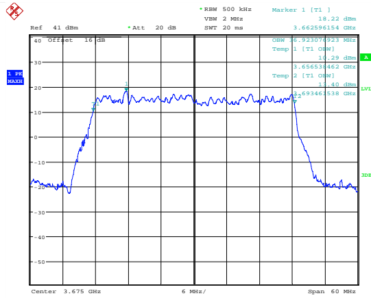
Date: 7.JUL.2018 19:50:09 99 % Bandwidth; QPSK; 3675 MHz; MIMO B.
