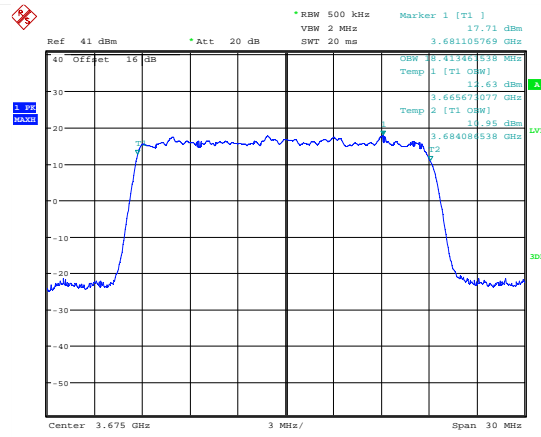
Date: 7.JUL.2018 17:01:49 99 % Bandwidth; QPSK; 3675 MHz; MIMO B.
