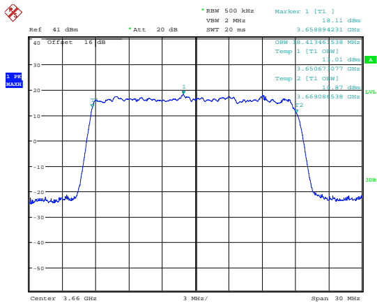
99 % Bandwidth; QPSK; 3660 MHz; MIMO A.
