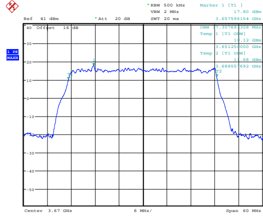
99 % Bandwidth; QPSK; 3670 MHz; MIMO B.
