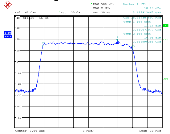
99 % Bandwidth QPSK; 3660 MHz; MIMO B.
