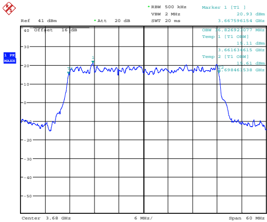
Date: 7.JUL.2018 20:22:33 99 % Bandwidth; QPSK; 3680 MHz; MIMO A.
