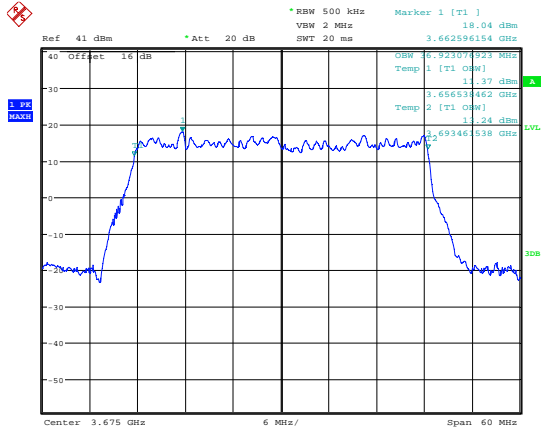
Date: 7.JUL.2018 19:52:56 99 % Bandwidth; QPSK; 3675 MHz; MIMO A.
