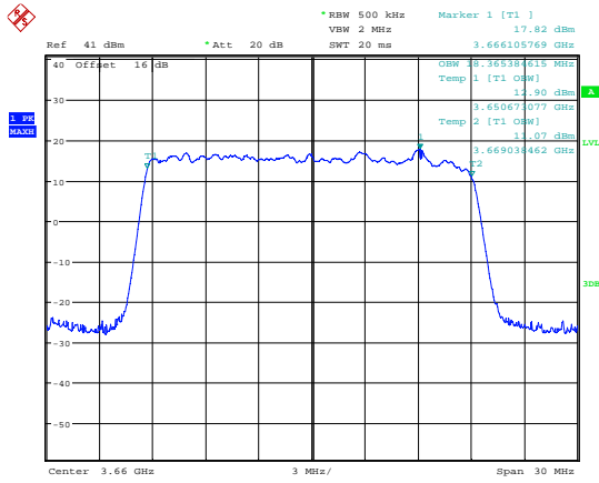
99 % Bandwidth QPSK; 3660 MHz; MIMO A.
