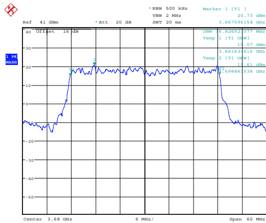
99 % Bandwidth; QPSK; 3680 MHz; MIMO B.
