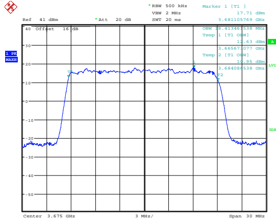
Date: 7.JUL.2018 17:01:49 99 % Bandwidth; QPSK; 3675 MHz; MIMO B.
