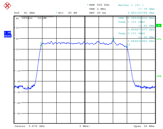
Date: 7.JUL.2018 17:11:45 99 % Bandwidth; QPSK; 3675 MHz; MIMO B.
