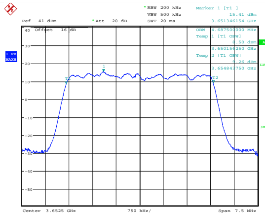
99 % Bandwidth QPSK; 3652.5 MHz; MIMO B.
