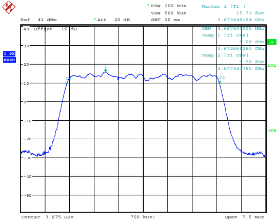
Date: 7.JUL.2018 18:50:33 99 % Bandwidth; QPSK; 3675 MHz; MIMO A.
