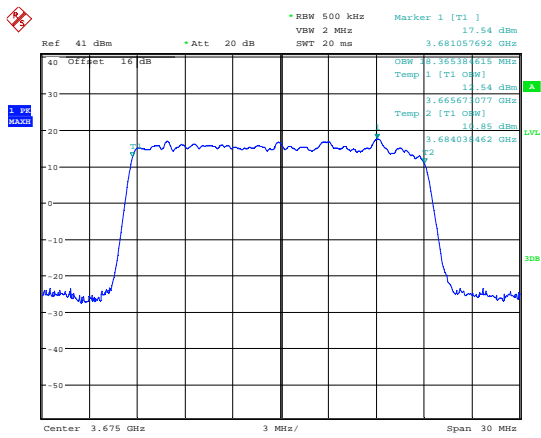
Date: 7.JUL.2018 17:18:05 99 % Bandwidth; QPSK; 3675 MHz; MIMO A.
