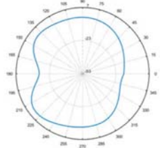
Total-Polar-E1-585MHZ
