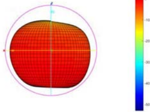
Total-3D-E1-585MHZ
