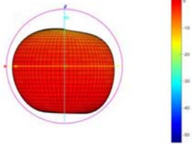
Total-3D-E1-600MHZ
