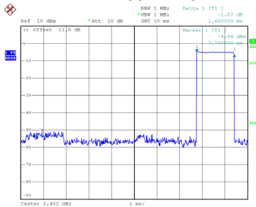
CH00-2DH3
