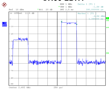
CH00-2DH1
