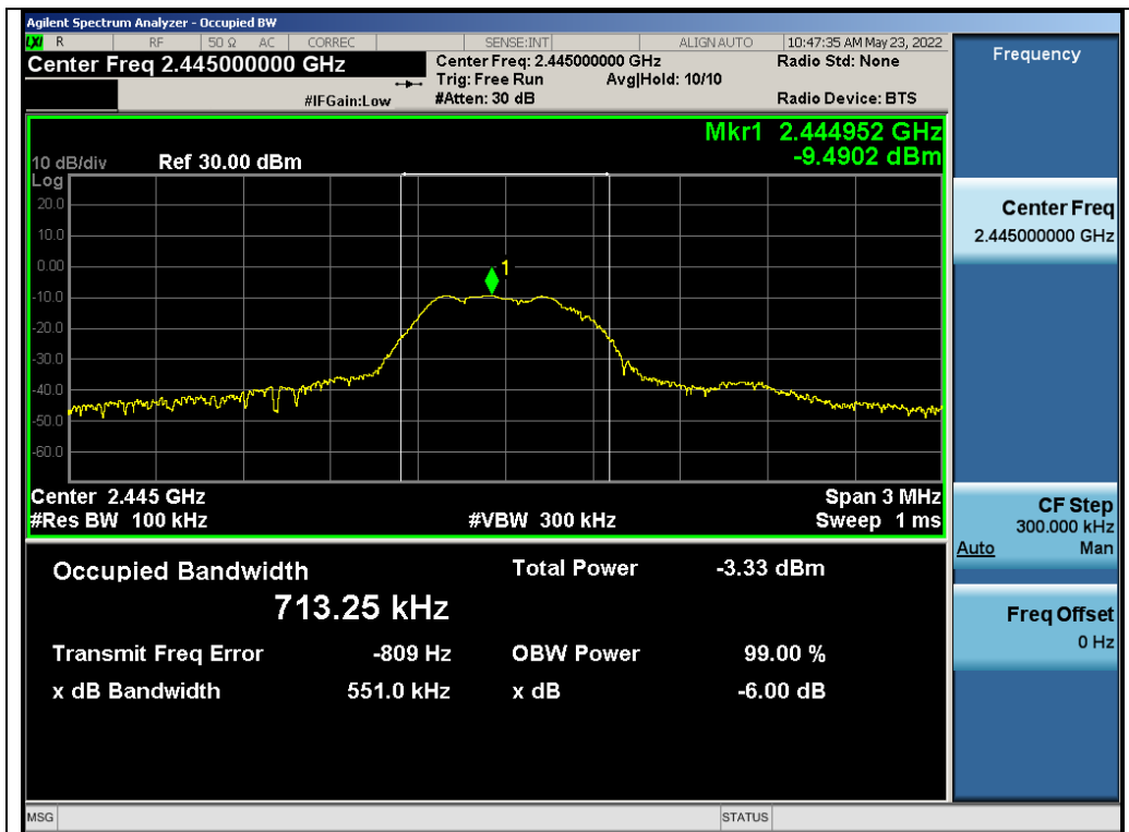
Test_Graph_GFSK_ANT1_2445_DTSBW
