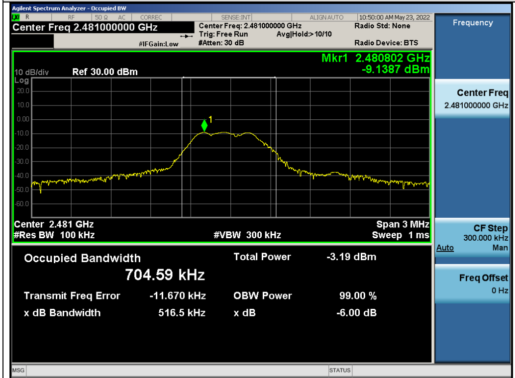
Test_Graph_GFSK_ANT1_2481_DTSBW
