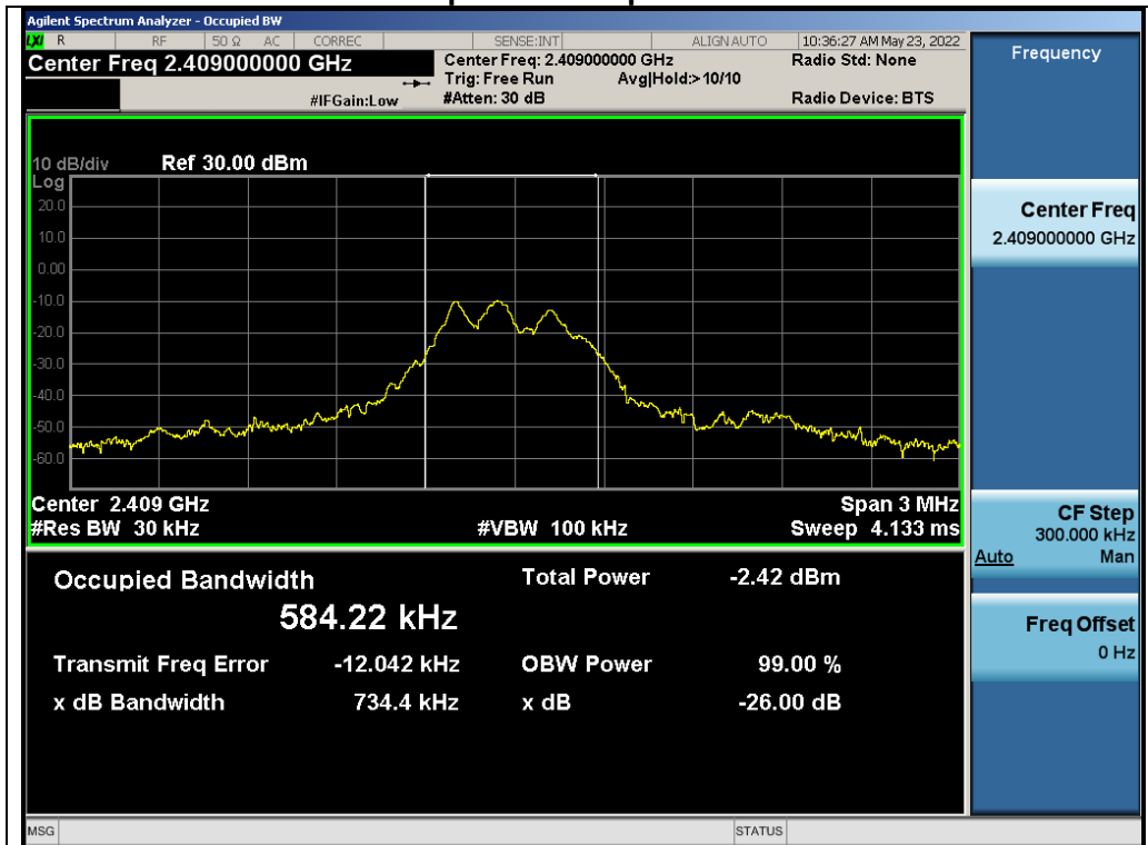
Test_Graph_GFSK_ANT1_2409_OBW
