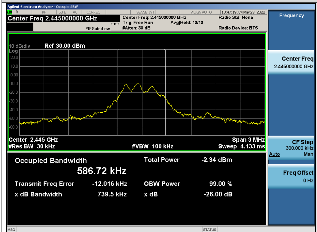
Test_Graph_GFSK_ANT1_2445_OBW
