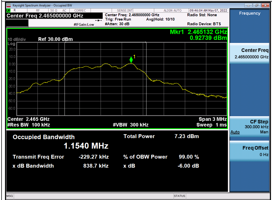
Test_Graph_GFSK_ANT1_2465_DTSBW
