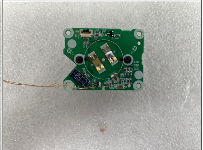
Antenna
