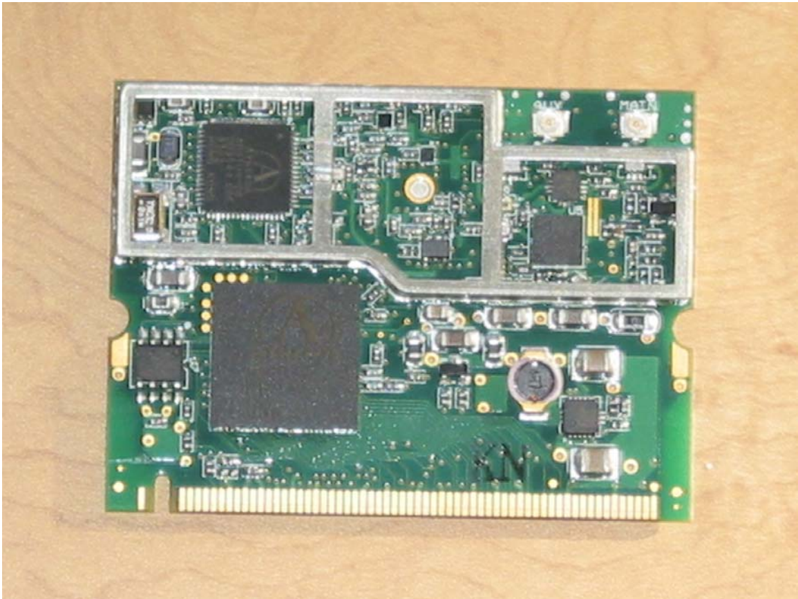
Mini PCI card, shield removed, Front
