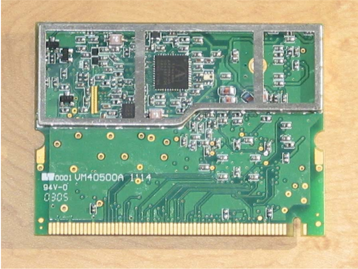
Mini PCI card, shield removed, Back
