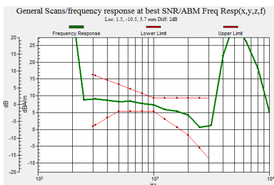
CDMA800 (BC0)
