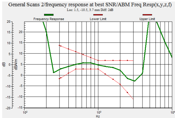
GSM850
