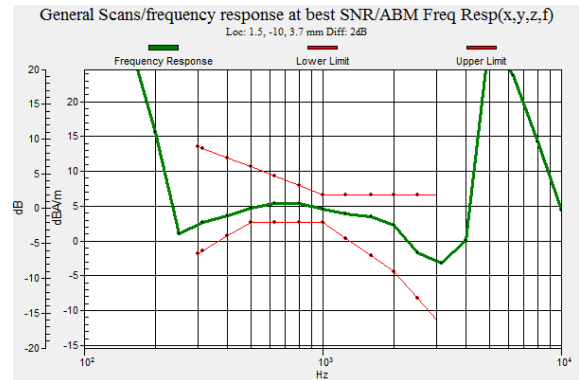
GSM1900
