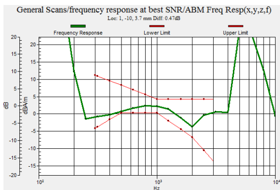
WCDMA850
