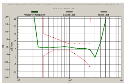
GSM850
