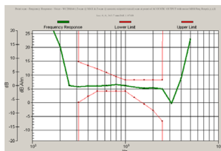
WCDMA1700/2100
