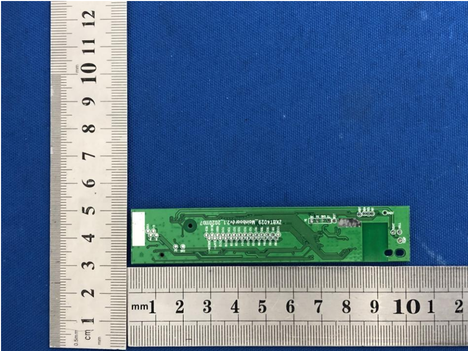
EUT Photo 18
