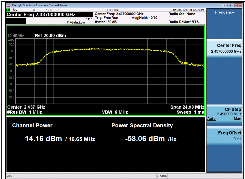
802.11g-2437MHz
