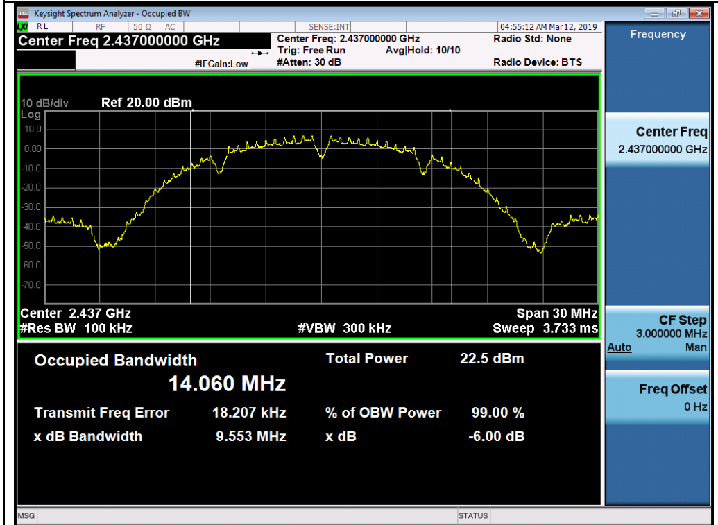
802.11b-2437MHz
