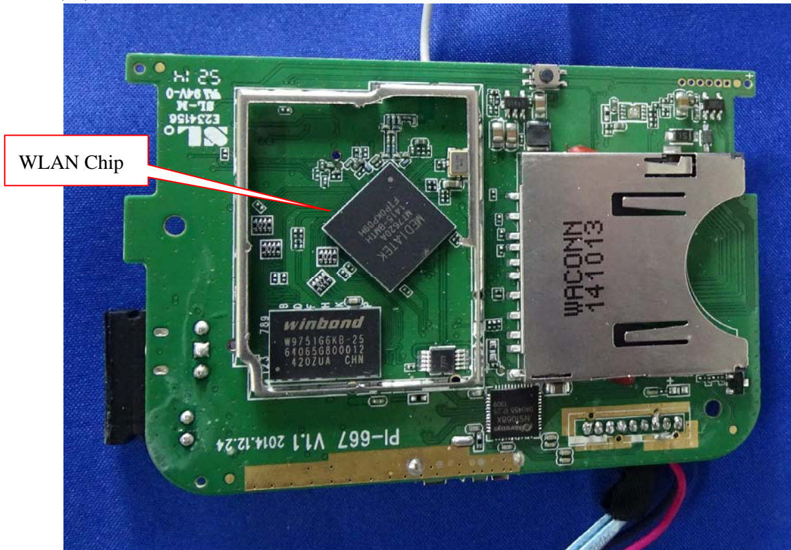
(16) EUT Photo
