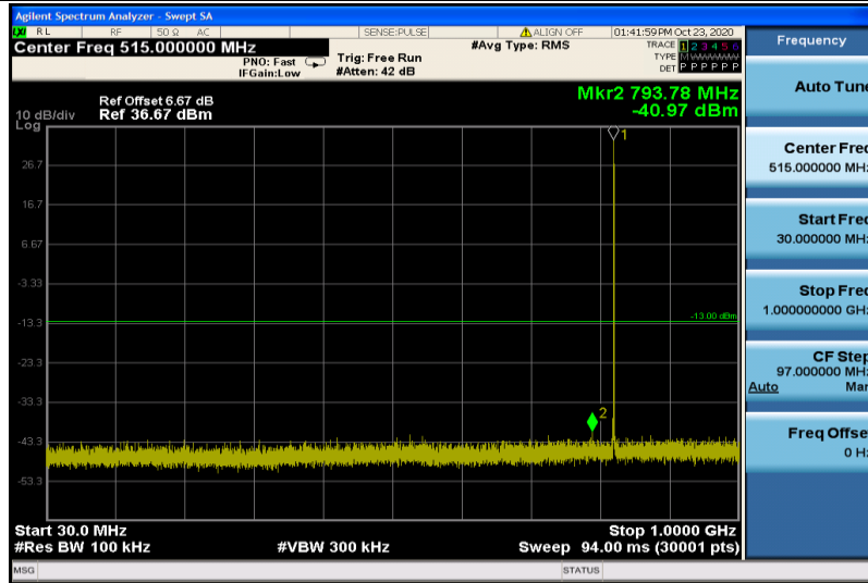
GSM850-128-30~1000
