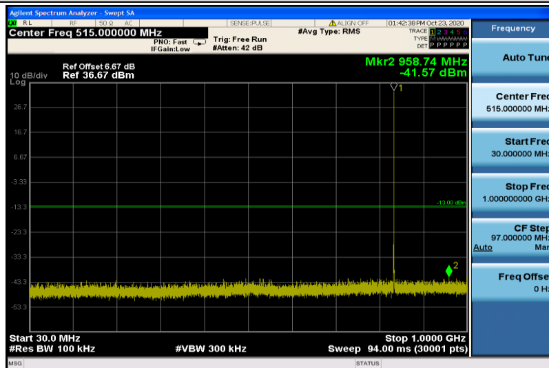
GSM850-190-30~1000
