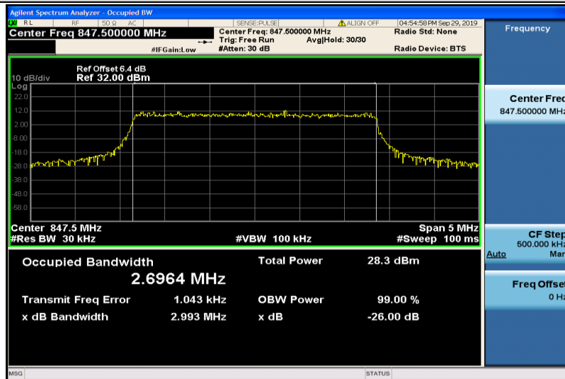
Band5-3MHz-QPSK-20635-15RB#0-2.6964
