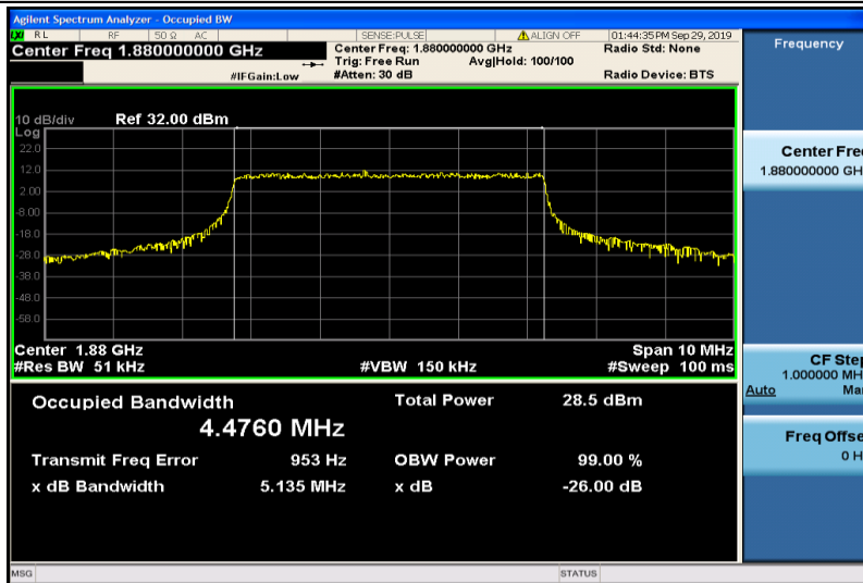
Band2-5MHz-QPSK-18900-25RB#0-4.4760
