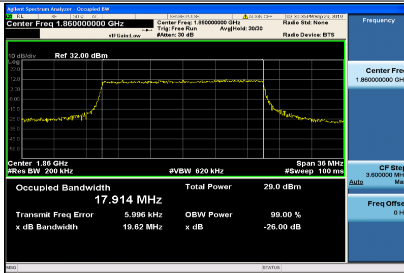
Band2-20MHz-QPSK-18700-100RB#0-17.914
