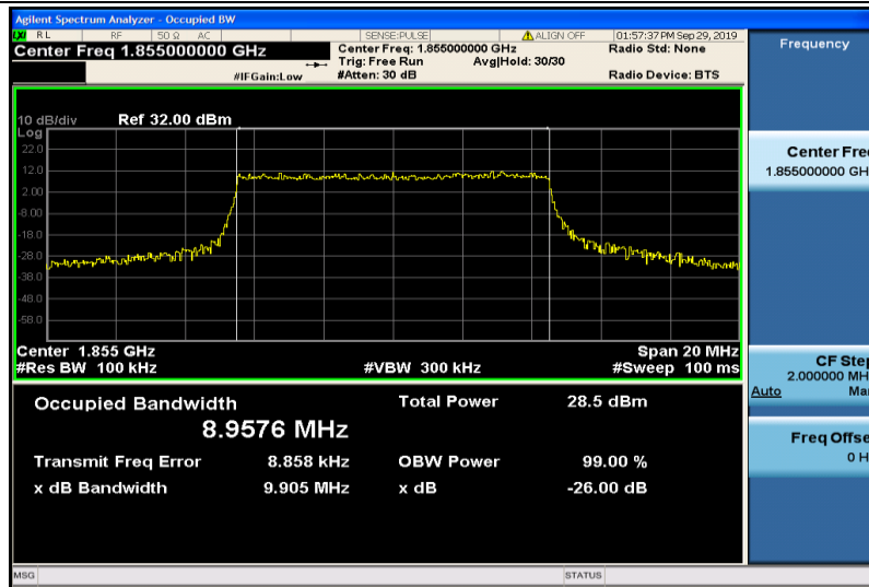
Band2-10MHz-QPSK-18650-50RB#0-8.9576
