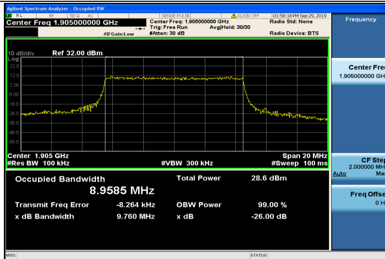
Band2-10MHz-QPSK-19150-50RB#0-8.9585
