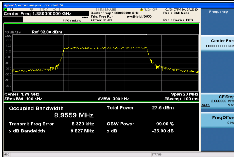
Band2-10MHz-16QAM-18900-50RB#0-8.9559
