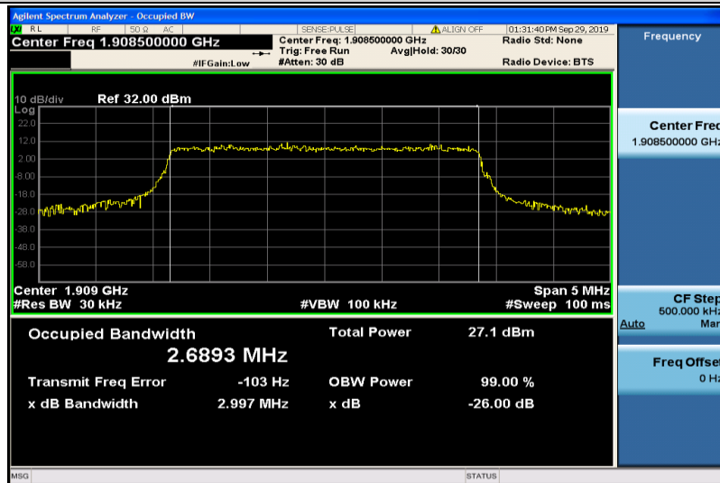
Band2-3MHz-QPSK-19185-15RB#0-2.6893
