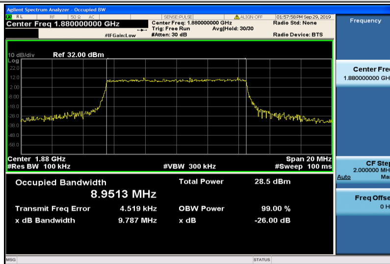
Band2-10MHz-QPSK-18900-50RB#0-8.9513
