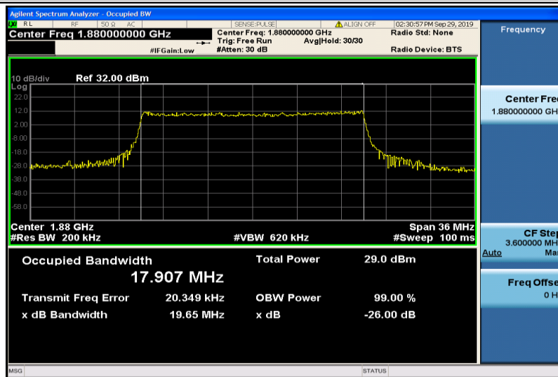
Band2-20MHz-QPSK-18900-100RB#0-17.907
