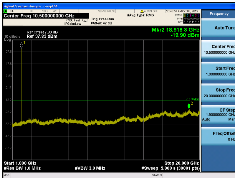
GSM1900-810-1000~20000
