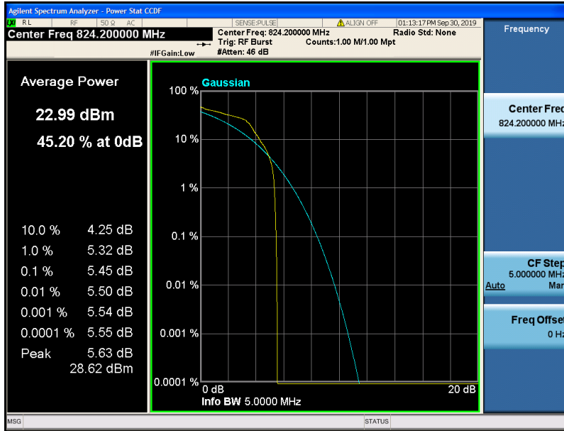
EGPRS850-128
