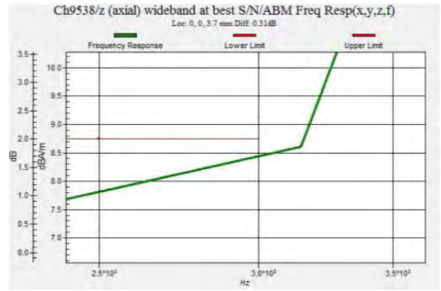
Fig. 7.18 WCDMA Band II Ch9538
