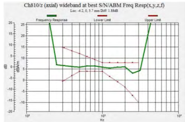
Fig 7.6 GSM1900 Ch810
