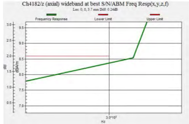
Fig. 7.10 WCDMA Band V Ch4182
