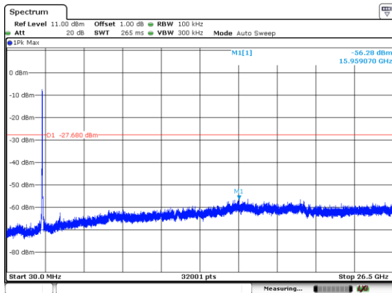
CH09-SE
