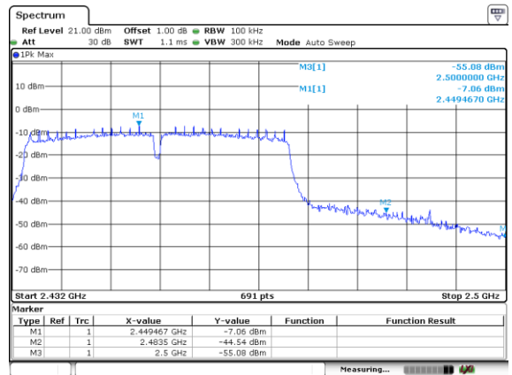
CH09-Bandedge
