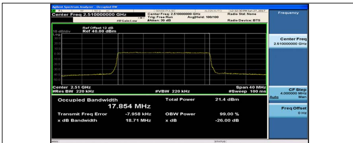
Band7_20MHz_16QAM_20850_100RB#0
