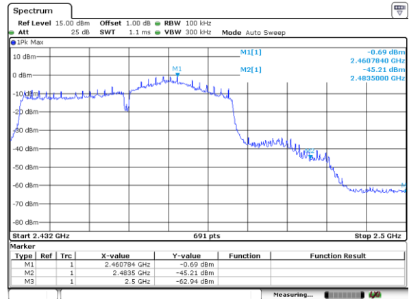
CH09-Bandedge
