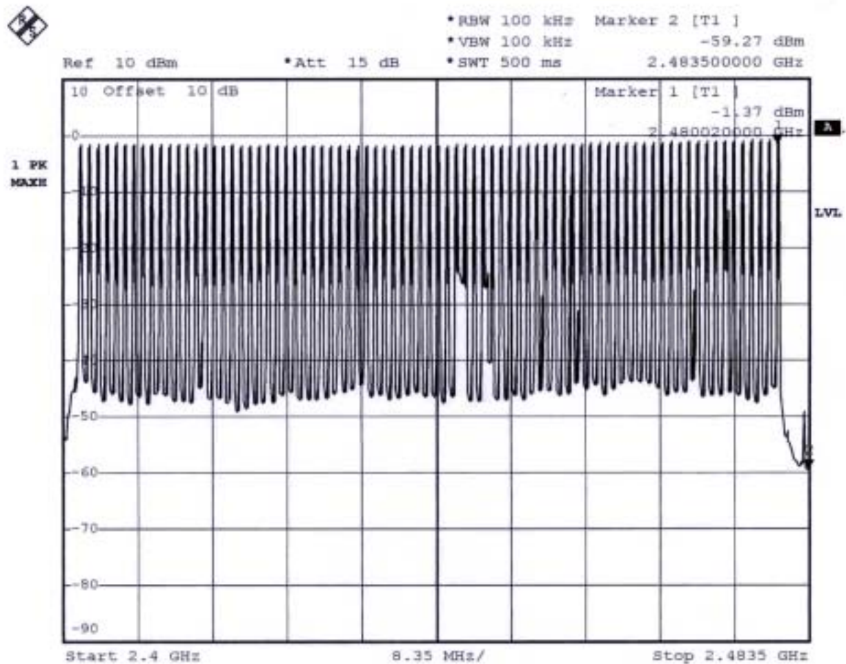
Plot 1 :
