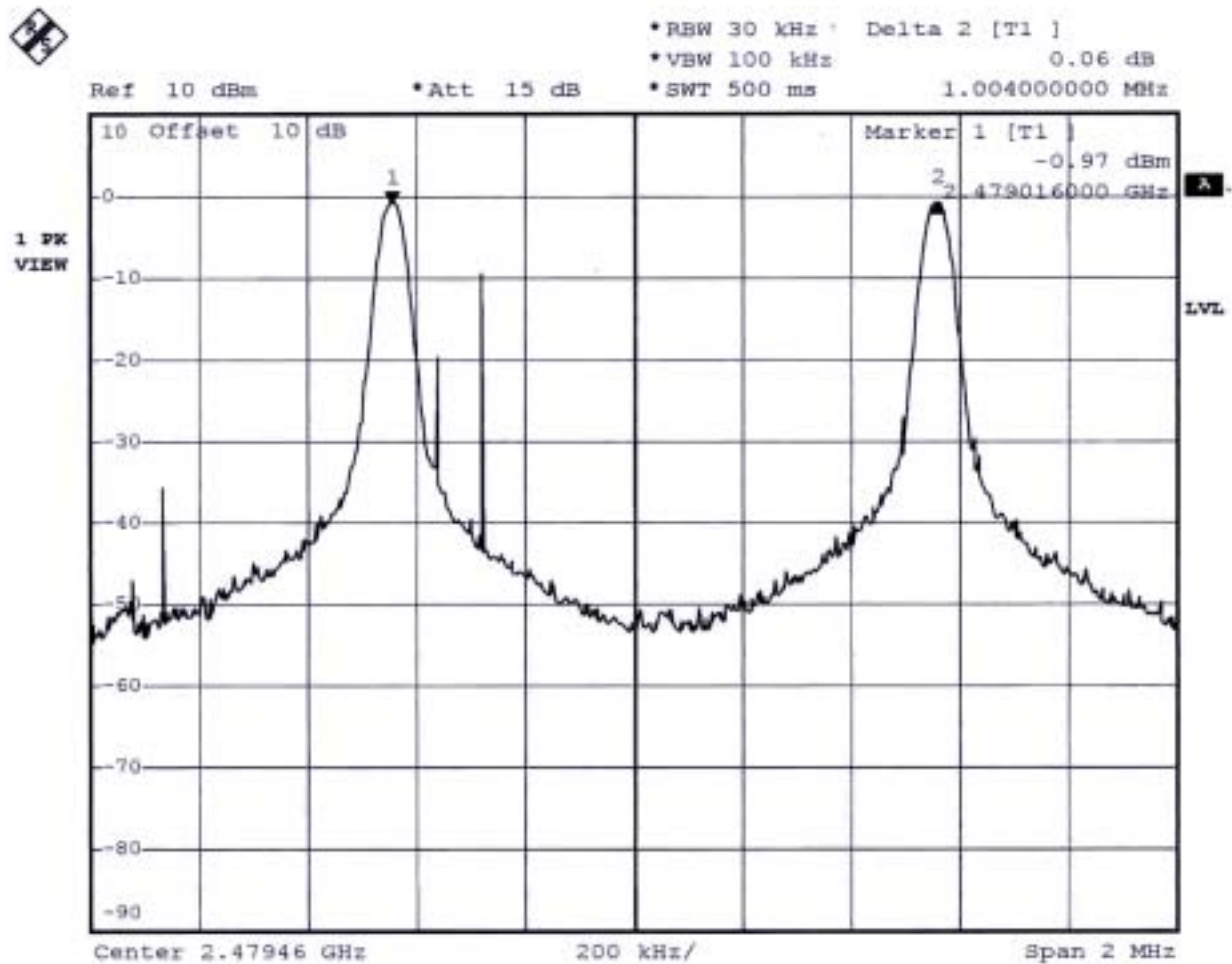
Plot 3 (Channel 78) :
