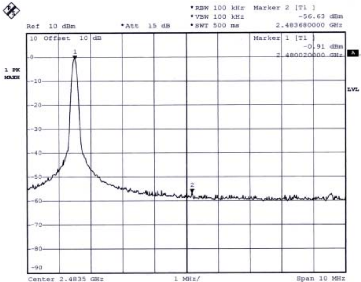
Plot 2 (Channel 78) :
