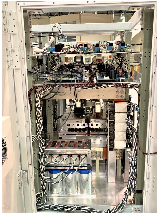
2 MVar. Module
