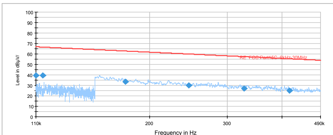
FCC RE 110K-490kHz AV
