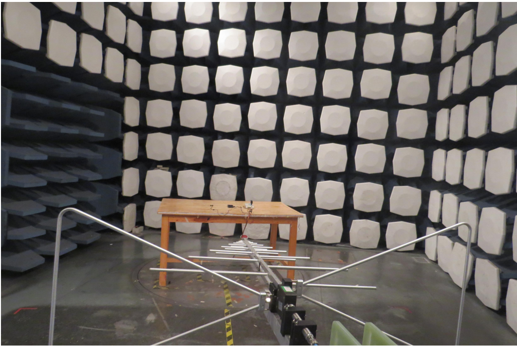
30MHz ~ 1GHz
