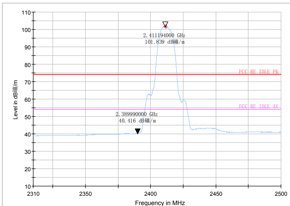
AV detector
