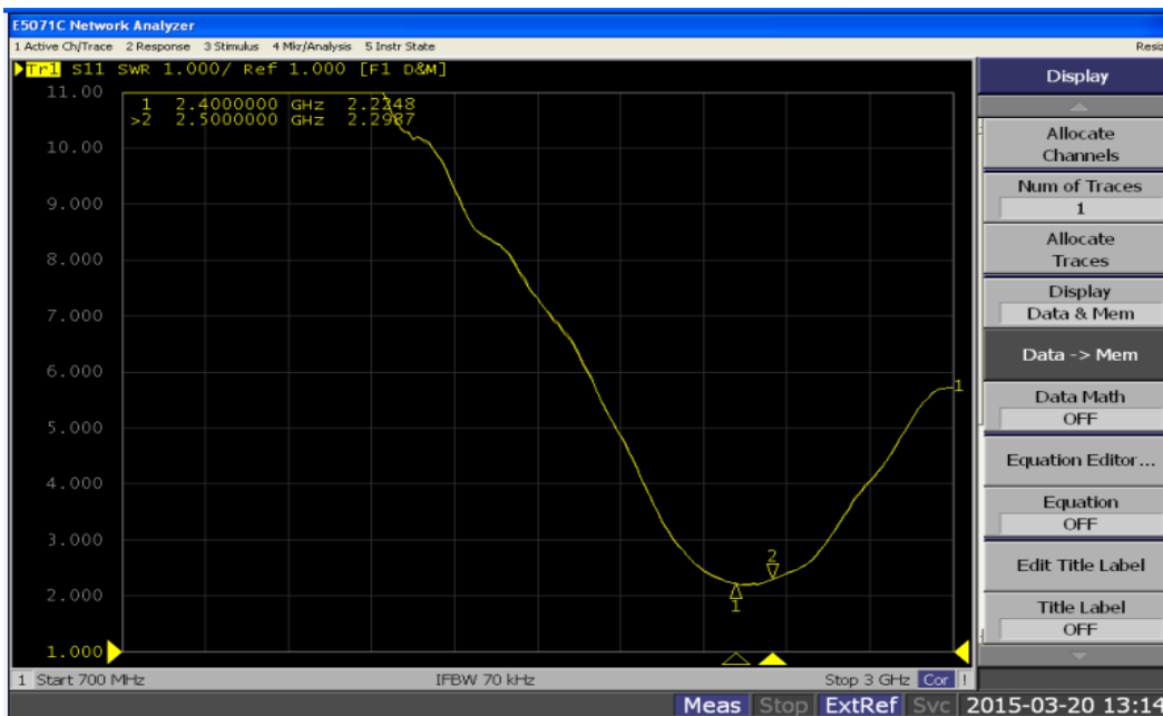
电压驻波比图
