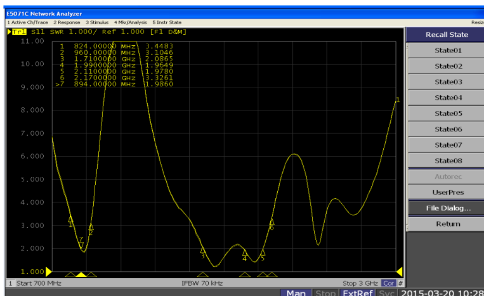
电压驻波比图
