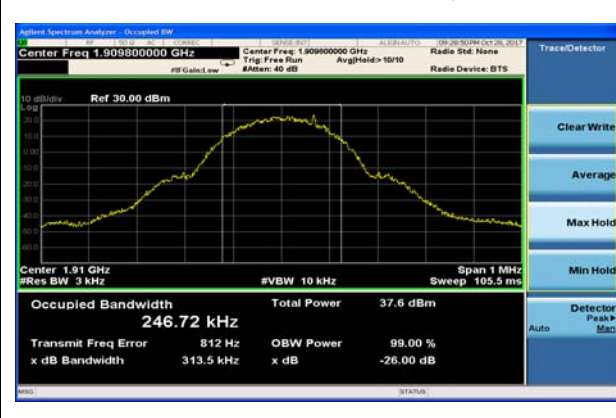
GSM 1900 GSM CH-High
