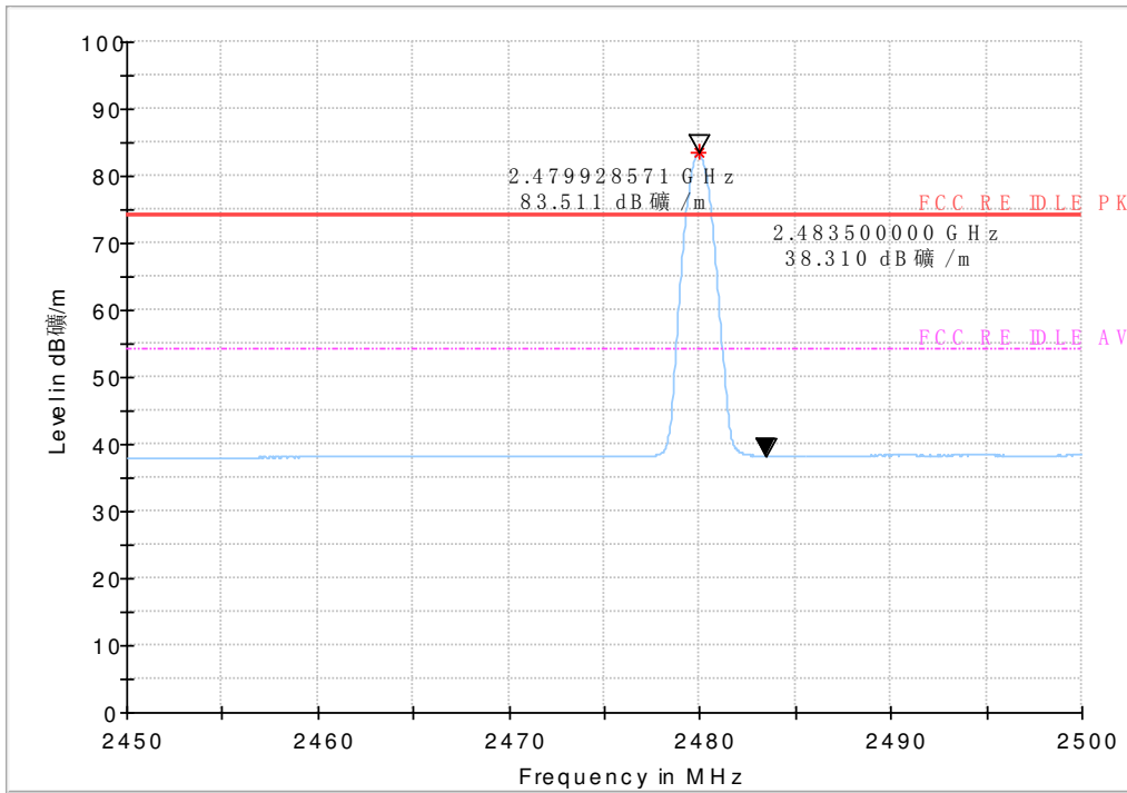
AV detector
