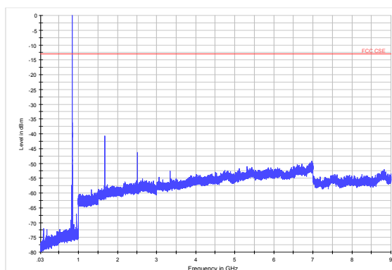
GSM 850 CH-High 30MHz ~ 9GHz
