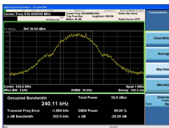
GSM 850 CH-Middle
