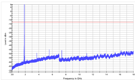
GSM 1900 CH-Middle 30MHz~18GHz
