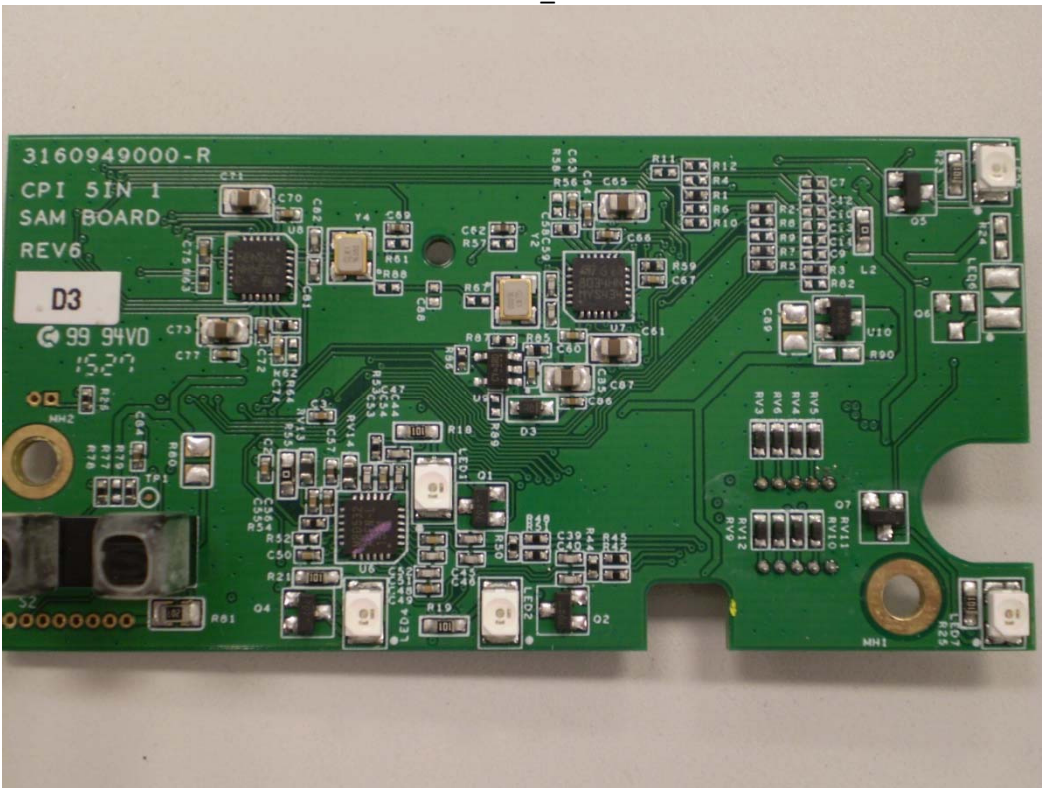
SAM PCB_Front
