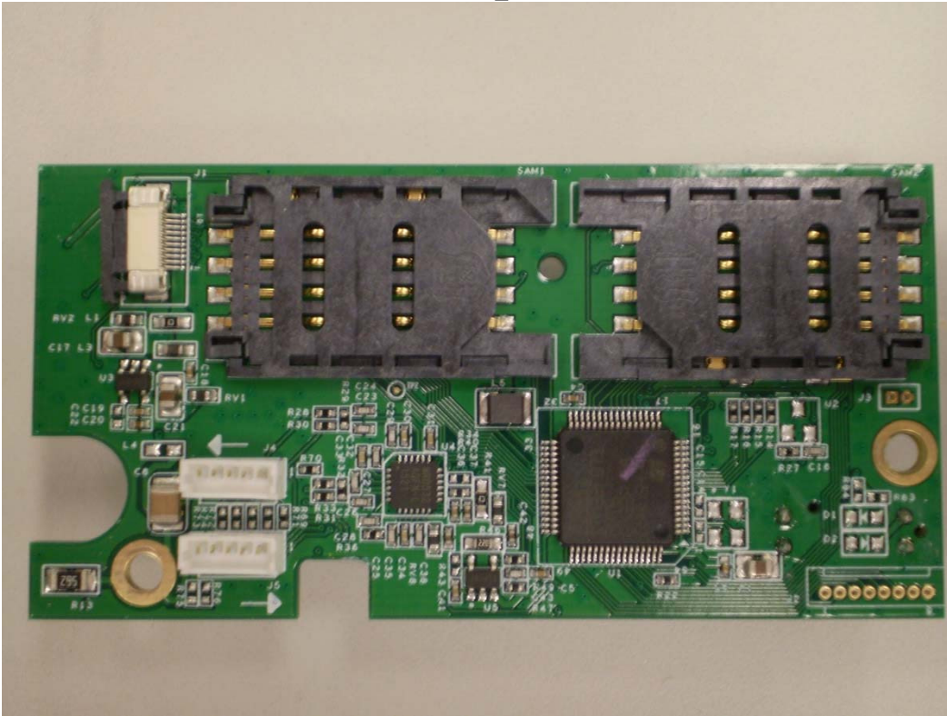
SAM PCB_Back
