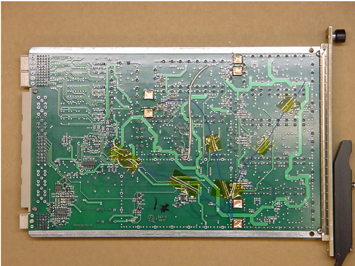
Photograph 9. LO Bottom
