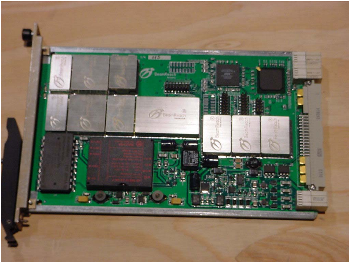
Photograph 21. PRBT Top
