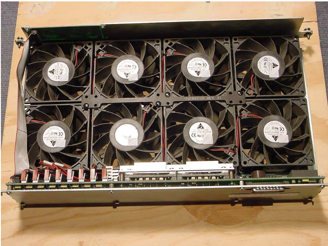
Photograph 4. Fan Tray Top
