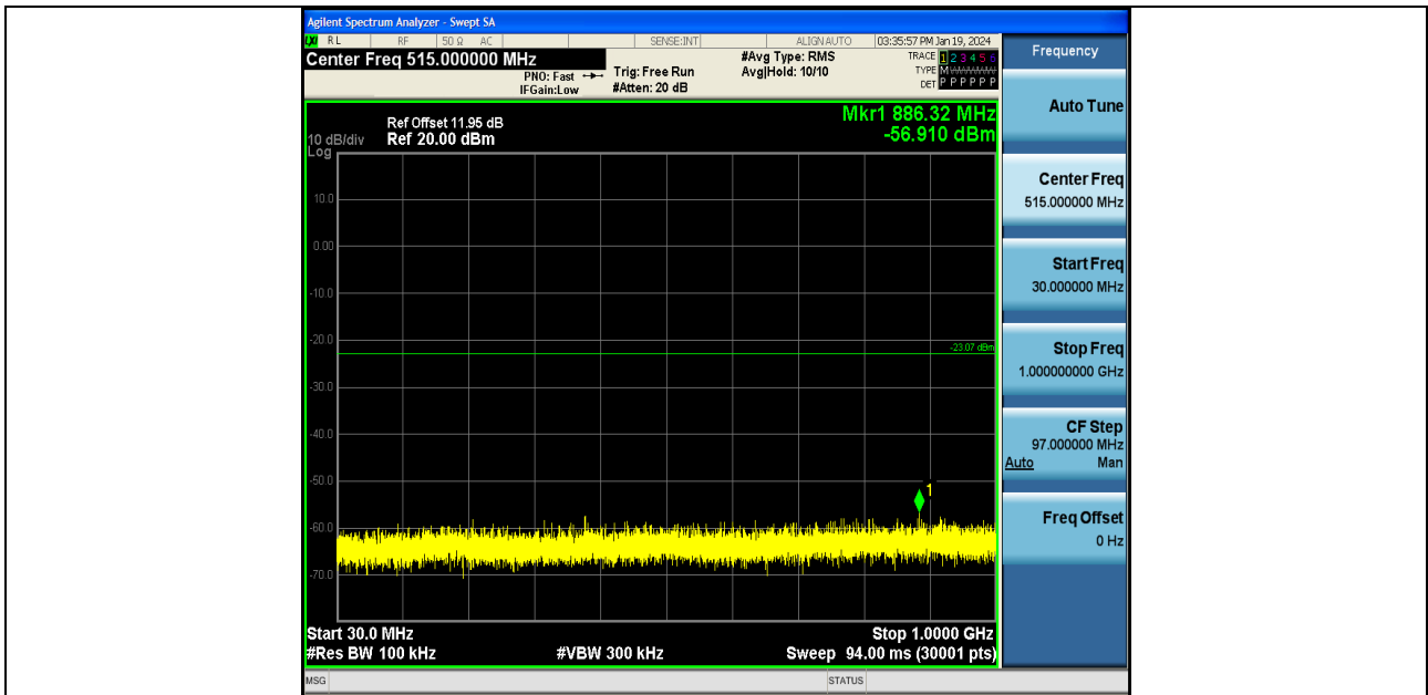
11G-Ant1-2412-30~1000-PASS
