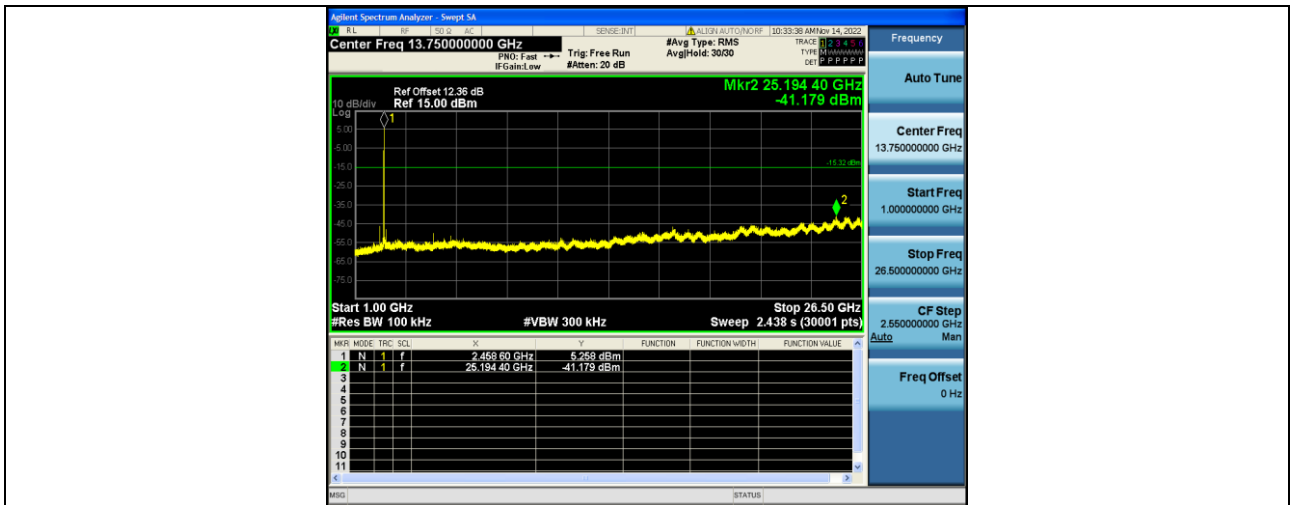
11G-Ant1-2412-0~Reference--5.07
