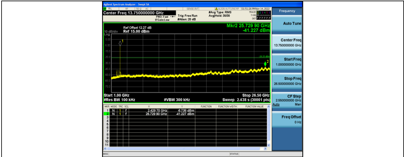
11N20SISO-Ant1-2462-0~Reference--7.47
