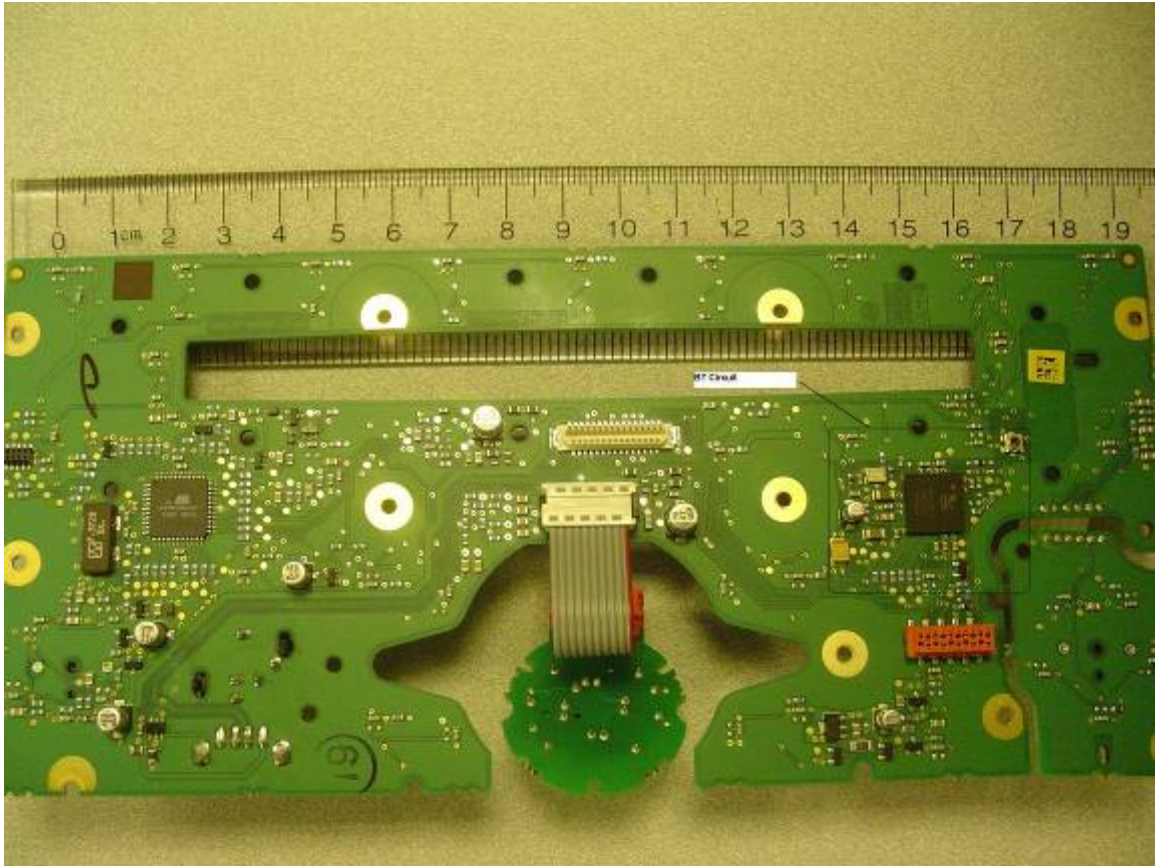
BT_Module_Back
