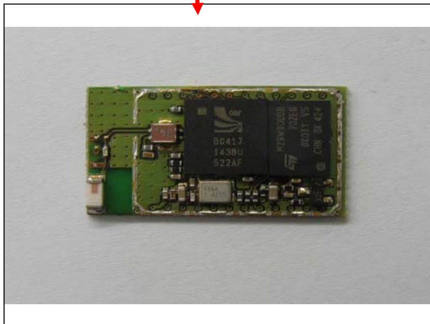
<BT Module>
