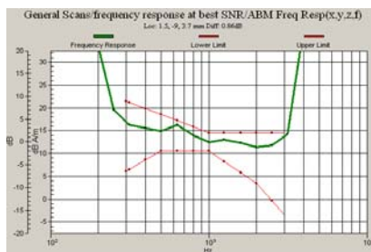
WCDMA1700/2100
