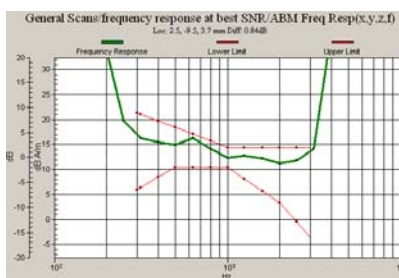
WCDMA1900
