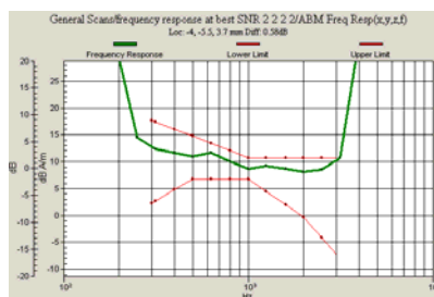
GSM1900
