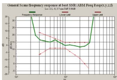
WCDMA850
