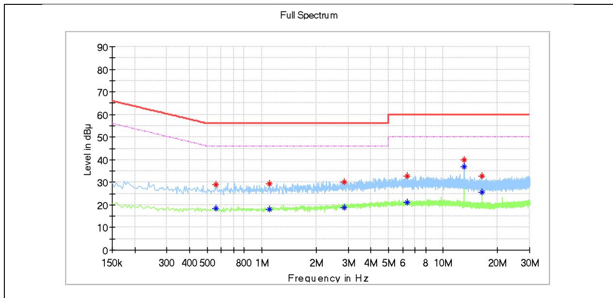
(L Phase)
