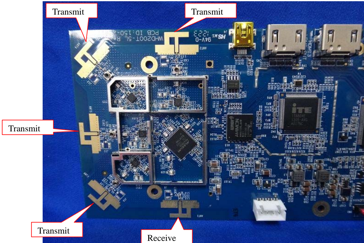
(12) EUT Photo (Antenna)
