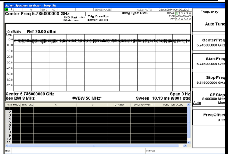
IEEE 802.11n-HT20
