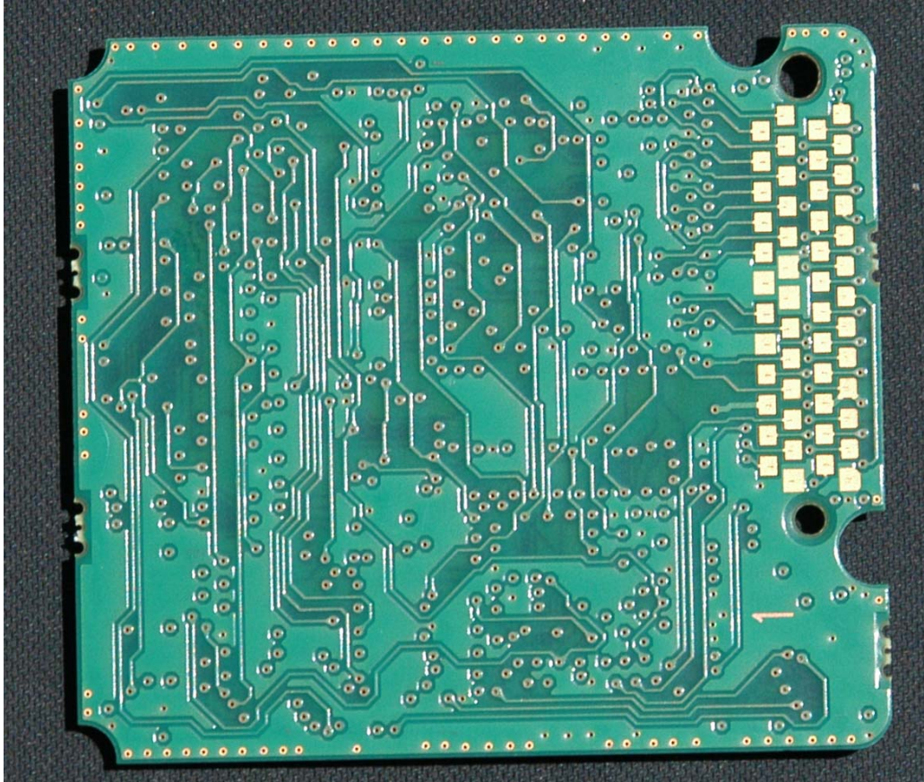
Vocoder board
