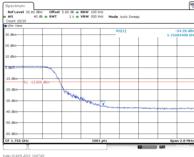
Band4_15MHz_QPSK_2025_1RB#0
