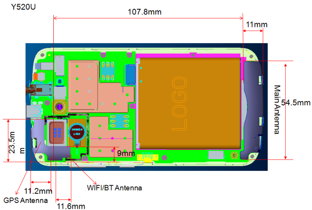
b: Antenna
