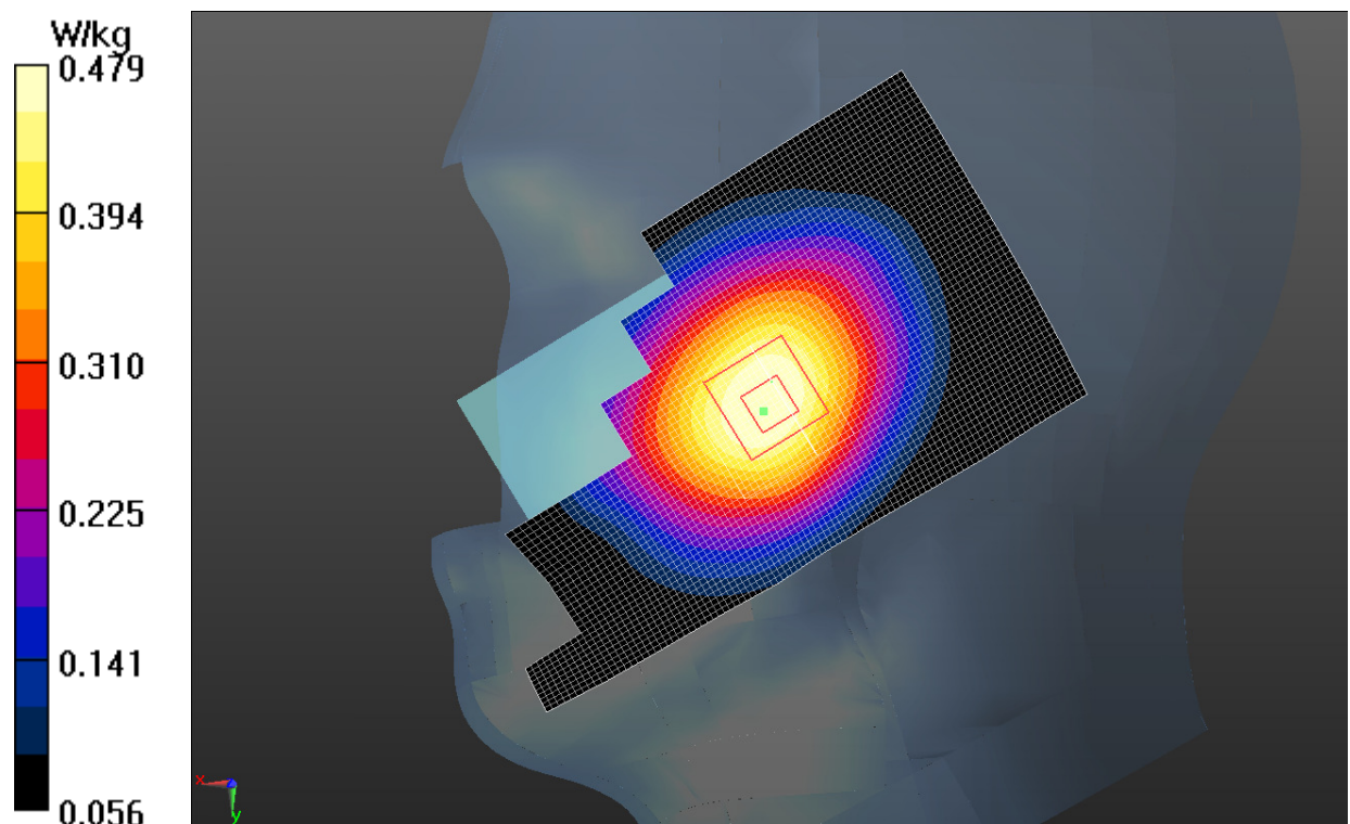
Fig.5 WCDMA 850
