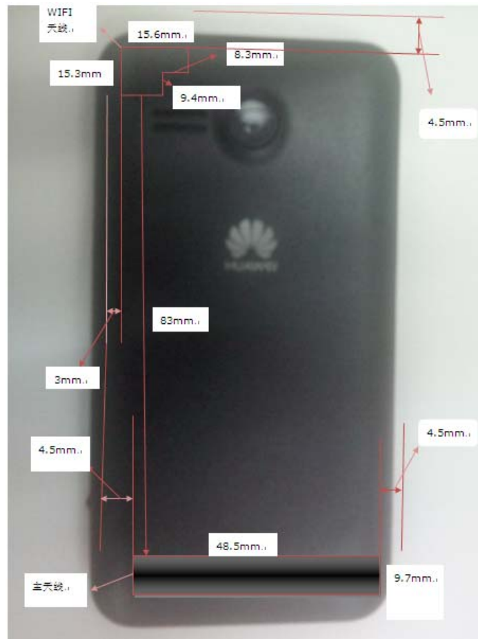
b: Antenna
