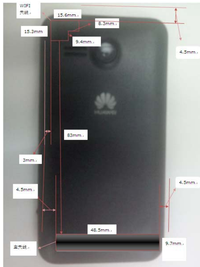
b: Antenna
