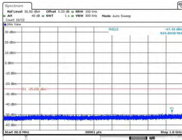
Band41_20MHz_QPSK_40640_1RB#0
