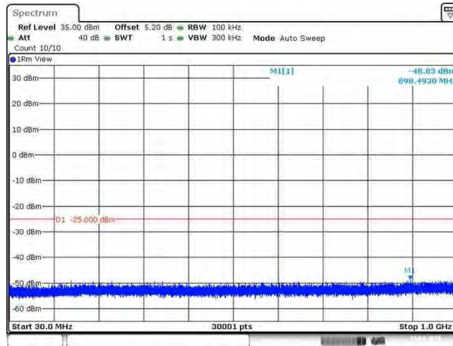
Band38_20MHz_QPSK_38150_1RB#0
