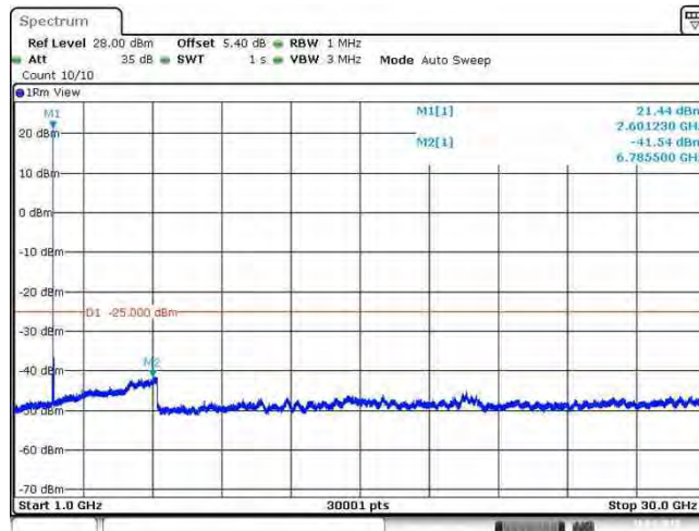
Band38_20MHz_QPSK_38150_1RB#0
